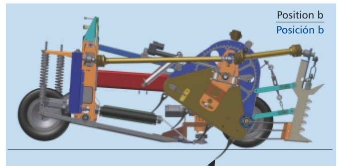
Platform auger positioned to lift the fallen plants forward. Posición del molinete que eleva las plantas derribadas hacia adelante.
