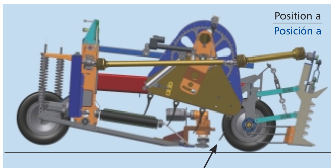
Normal platform auger position. Posición normal del molinete
